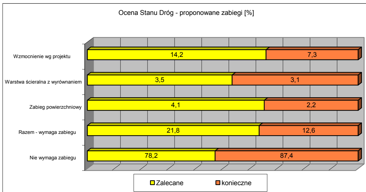
Rysunek nr 4. Zabiegi zalecane i konieczne, proponowane do wykonania na drodze nr 4
