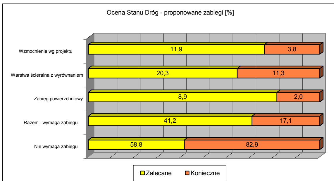
Rysunek nr 8. Zabiegi zalecane i konieczne, proponowane do wykonania na drodze nr 8
