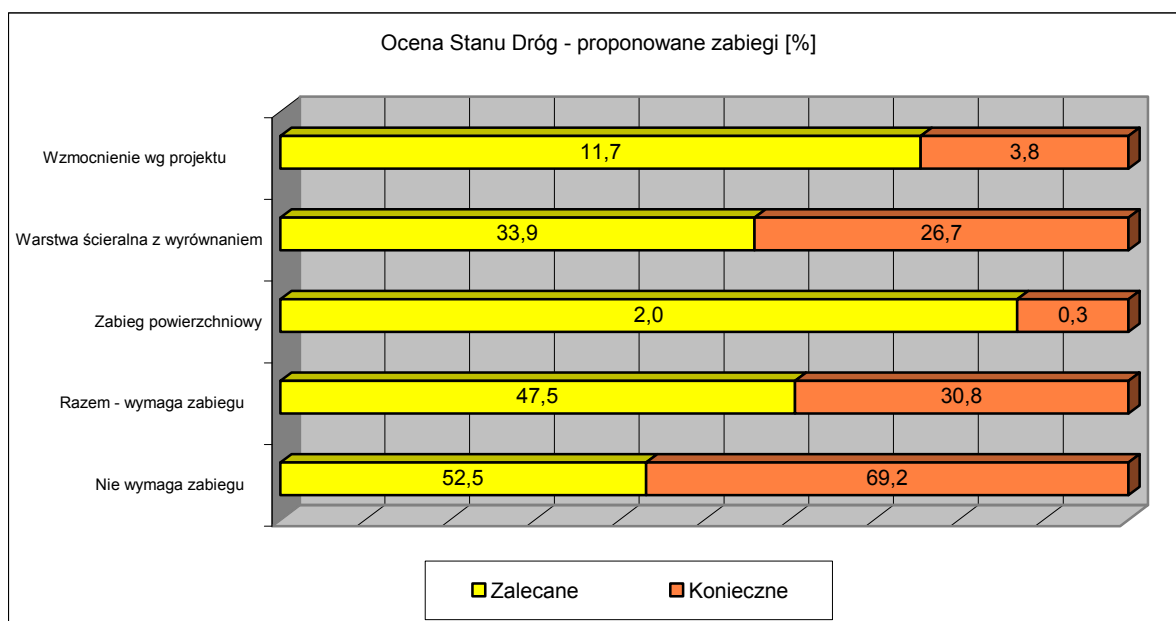
Rysunek nr 13. Zabiegi zalecane i konieczne, proponowane do wykonania na drodze nr 16
