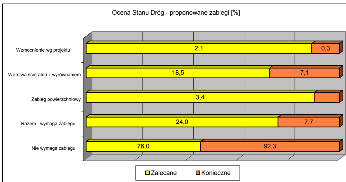
Rysunek nr 6. Zabiegi zalecane i konieczne, proponowane do wykonania na drodze nr 6
