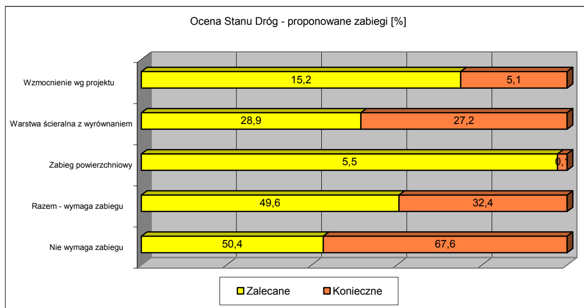
Rysunek nr 12. Zabiegi zalecane i konieczne, proponowane do wykonania na drodze nr 12
